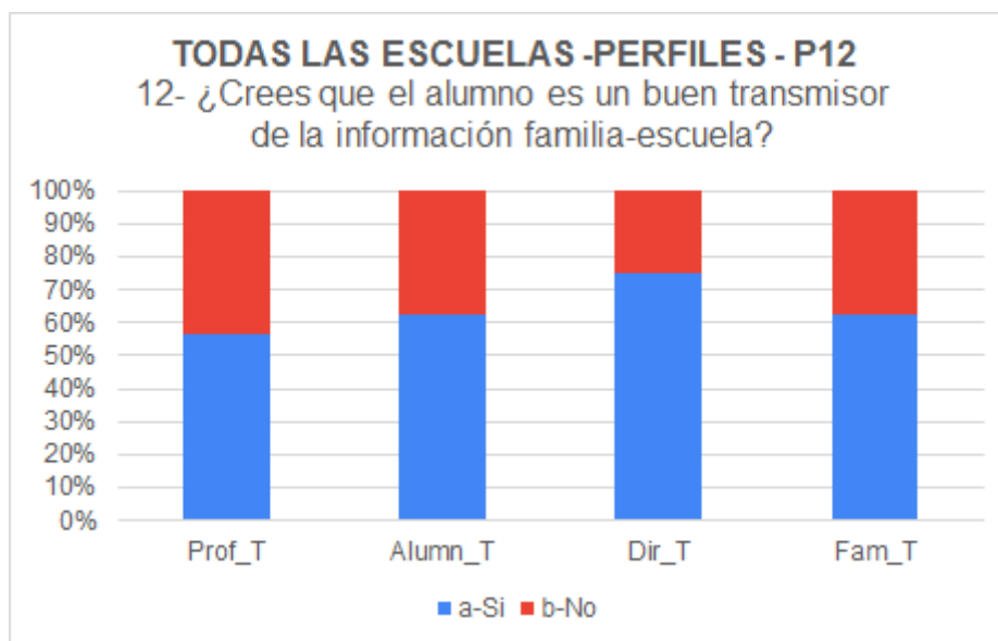
[Fig. 6]- Porcentaje de respuestas de cada sector educativo indicando si consideran al alumnado un transmisor fidedigno de información.
