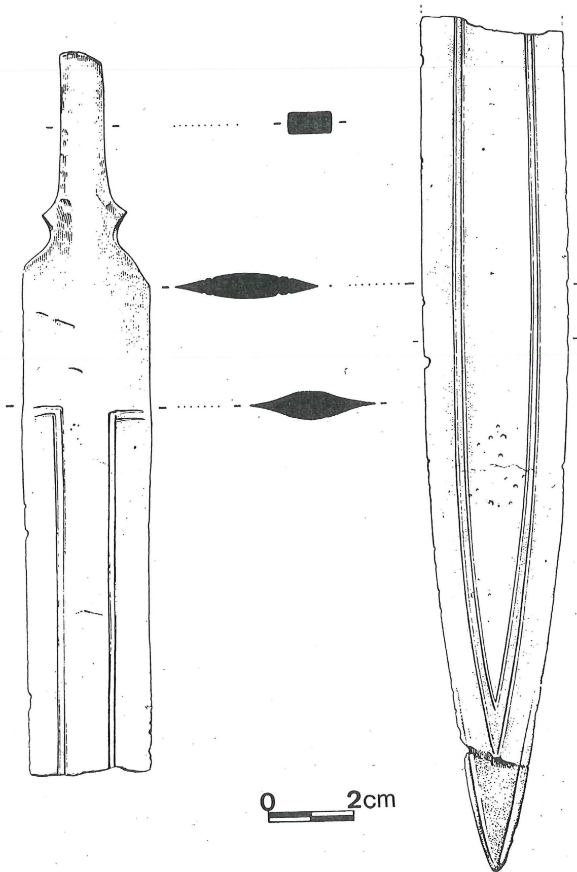
Fig. 4.—Espada relacionada con el “tipo Monza”, procedente de La Llacura (Barcelona) (según J. M. Masach).
