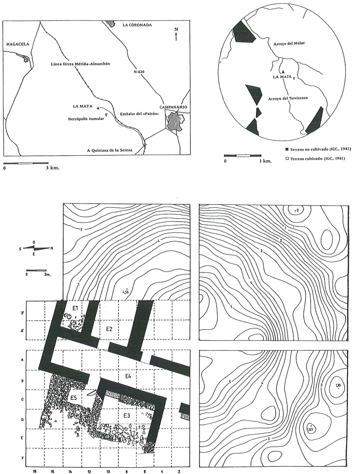
Figura 1. Planta-croquis de La Mata de Campanario (Badajoz) (1990-1994).
