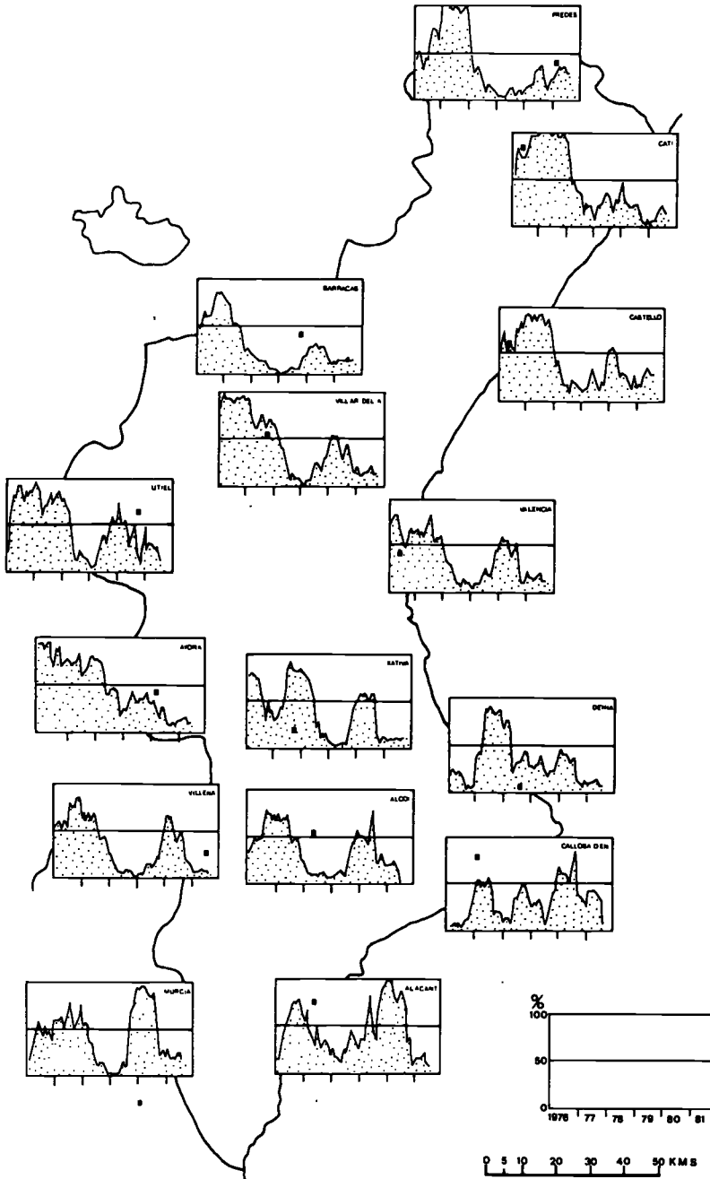
Figura 2.—Distribución espacial de la evolución de probabilidades de recurrencia de periodos de doce meses.
