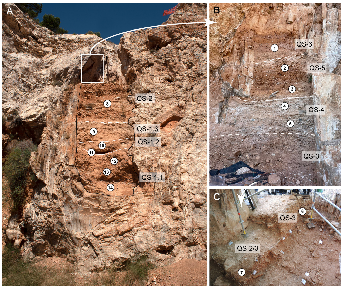
Figura 3. Puntos de muestreo en la sección de Quibas-Sima. A , Muestras 8–14 del perfil estratigráfico original (unidades QS-1 y QS-2); B , muestras 1–5 del perfil testigo de la sección (unidades QS-6 a QS-4); C , muestras 6 y 7 de la superficie de excavación (unidades QS-3 y QS-2/3).
